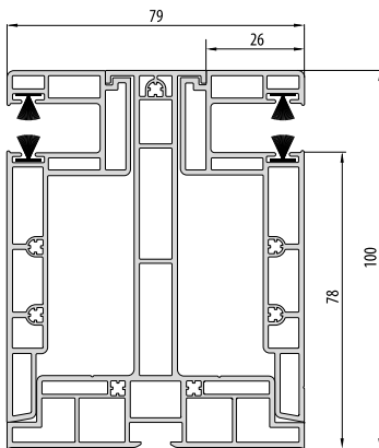
• PPDRA 79 • Styroterm Revision von außen
