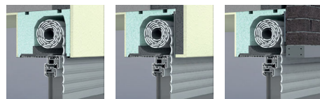
Monolithischer Putz
