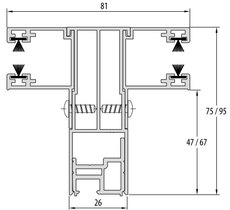
• Teilungsschiene RGT 75/95 • Roka top 2 RG / RG EX
