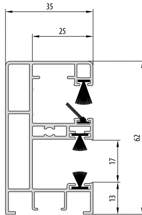
• PPAM 35/17* • Opterm
