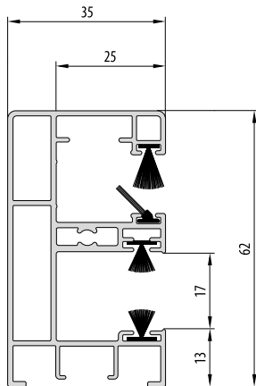
• PPAM 35/12* • Opterm
