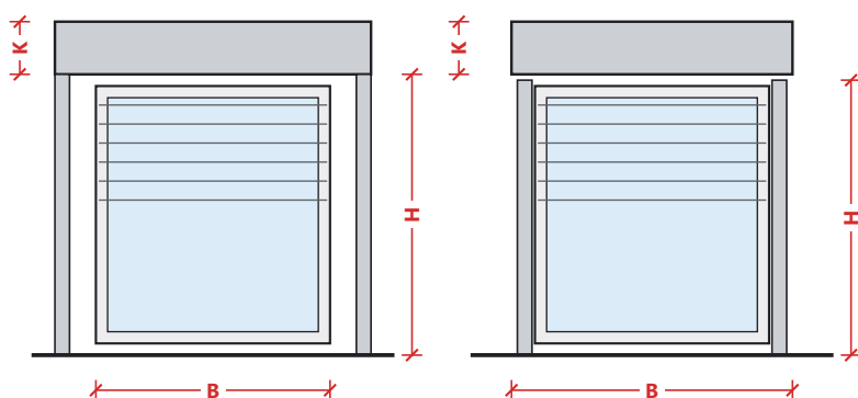
Vorbaujalousie
